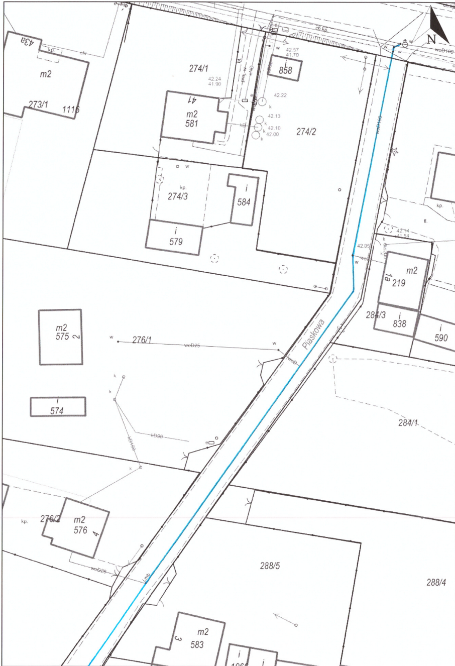
Wydruk w skali 1:500
