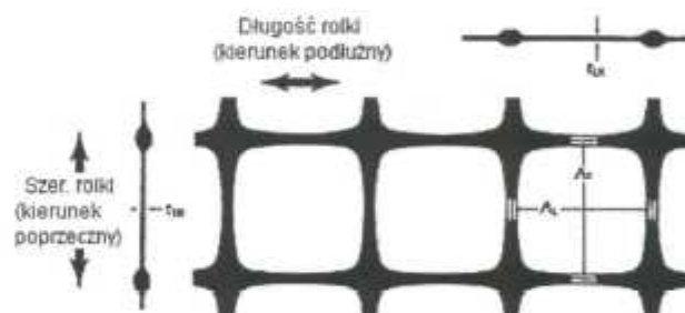
Rys. 2. Struktura georusztu typu Tensar SS-40
