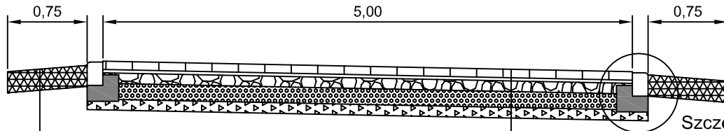
Szczegół "A"
